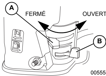
Figure 3-2. Robinet de carburant et levier d'étrangleur
