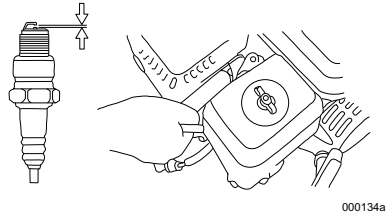
Figura 4-8. Bujía
